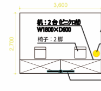
■出店ブース (物販) 詳細図 (scale=1/100)
