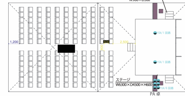
■ステージ拡大図 (scale=1/150)
